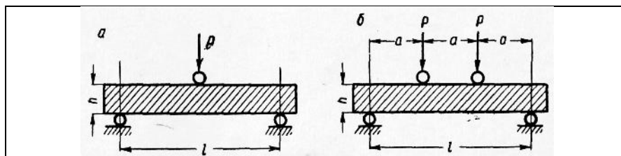
Рис. 1. Схемы испытания строительных материалов на изгиб сосредоточенными грузами: а - одним; б - двумя.
