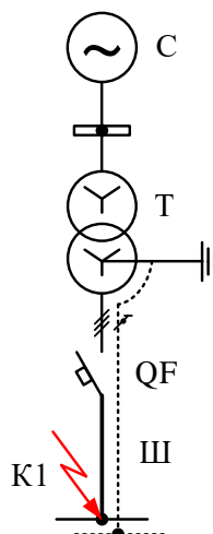
Рисунок 1. Схема сети.
