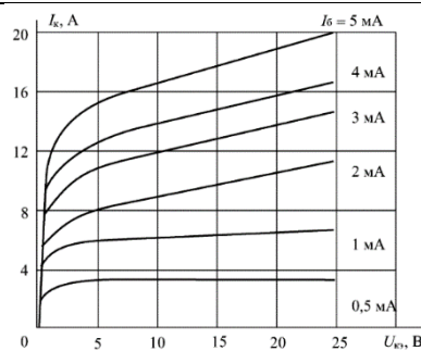
б. Выходные характеристики
